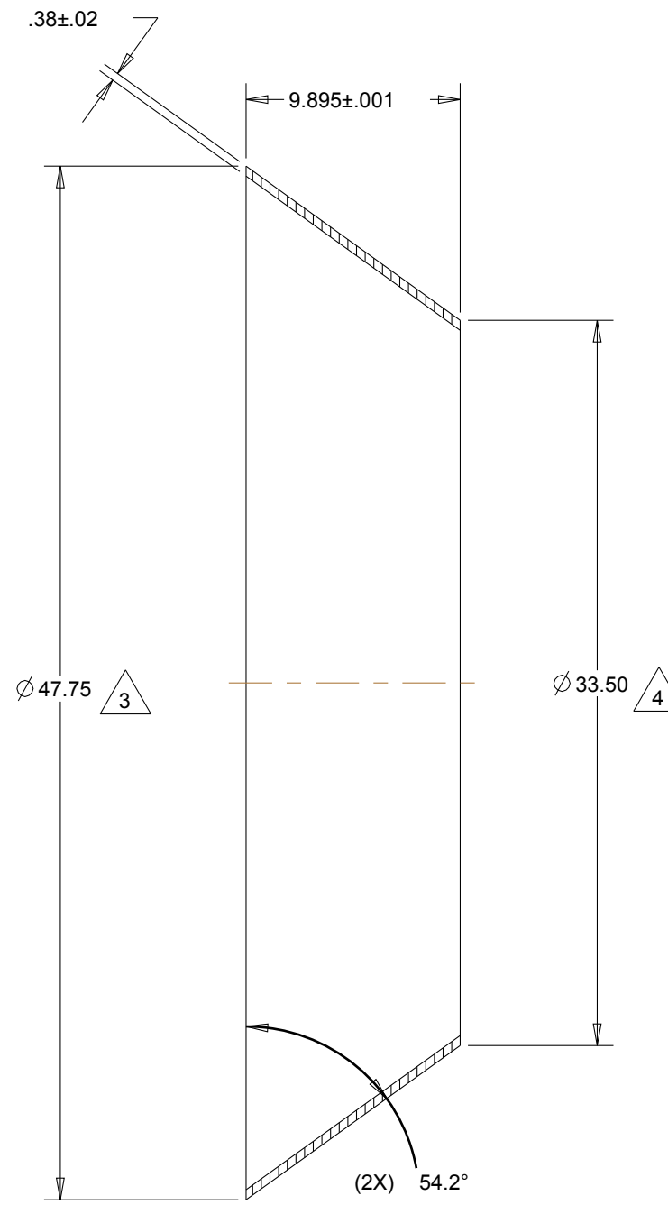
SECTION A-A
