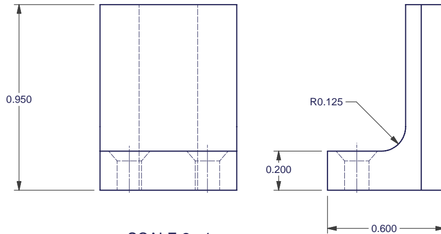
SCALE 2 : 1
